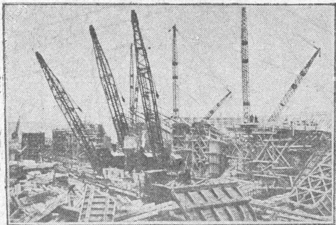
Днепрострой. Общий вид работ в котловане гидроэлектростанции
