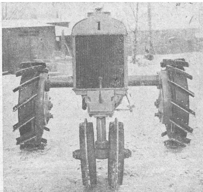
Пропашник конструкции инж. А. Г. Шевело
