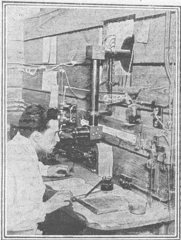
Лаборатория академика Павлова. Наружная стена звуко- непроницаемой камеры. Сотрудник наблюдает через перископ за собакой, находящейся внутри камеры
