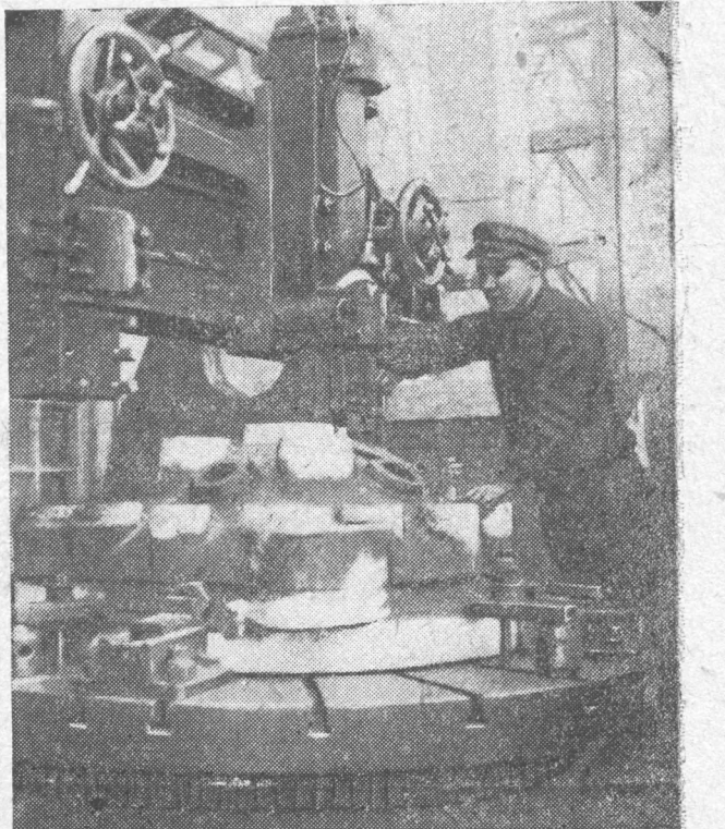
Завод „Русский дизель“. Обточка техмассовцем крышки дизеля на карусельном станке
